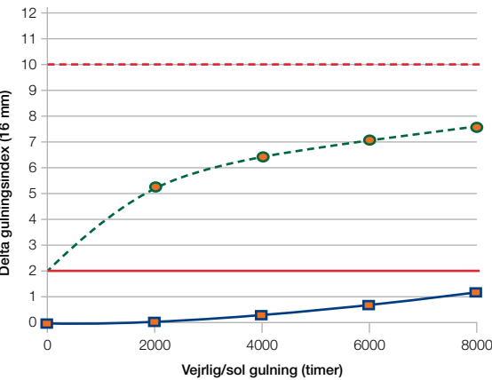
Gulingsindex. Data fra ATLAS Ci5000 (ISO 11341 / ASTM G155) om vejrlig.
