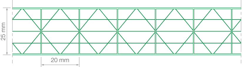
25 mm/5 lag/X struktur
